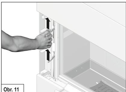
Obr. 11 Vytáhněte obě uzavírací západky (vlevo nebo vzpravo) směrem nahoru (obr. 11).
