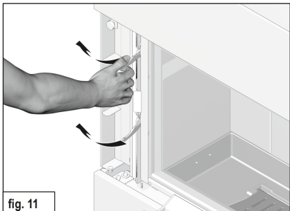
fig. 11 Ruotare a destra o a sinistra lo sportello della camera di combustione in corrispondenza della linguetta della maniglia (fig. 11).
