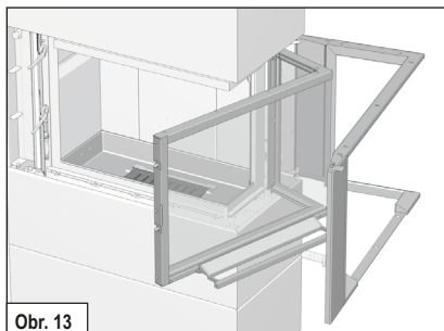
Obr. 13 Otevřená dvířka topeniště s otevřenými menšími dvířky dvířek topeniště (obr. 13).
