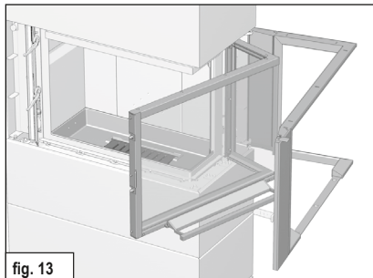
fig. 13 Lo sportello della camera di combustione con schermo di protezione aperto. (Fig. 13).
