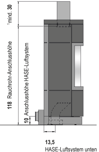
Seitenansicht LIMA C.16 / SILA:
